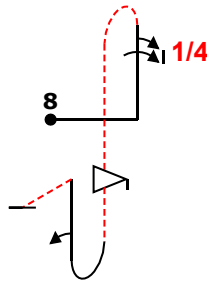
Fig H 8.8.5.1(21) 9.1.1.5(14) 9.9.10.4(13) 9.1.1.2(8) K: 56
