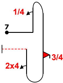
Fig G 8.8.1.1(18) 9.1.1.1(6) 9.10.10.3(15) 9.4.1.2(9) K: 48
