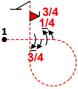
Fig A 8.6.7.4(16) 9.1.3.7(11) 9.1.3.5(9) 9.10.1.3(17) K: 53
