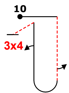
Fig J 8.4.4.3(14) 9.1.5.2(4) 9.4.1.3(12) K: 30
