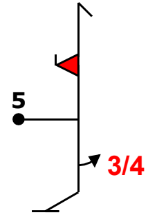
Fig E 5.2.1.1(17) 9.10.6.2(19) 9.1.5.3(6) K: 42
