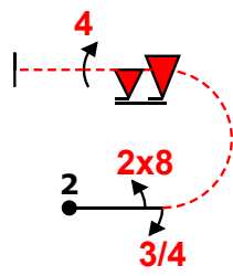
Fig B 7.2.4.1(8) 9.8.3.1(3) 9.1.3.3(6) 9.10.3.6(16) 9.4.3.4(11) K: 44
