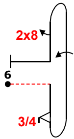
Fig F 8.8.1.4(18) 9.9.5.3(11) 9.1.1.4(12) 9.8.5.1(3) K: 44
