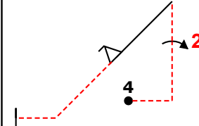
Fig D 1.2.7.2(17) 9.2.1.4(13) 9.9.4.2(11) K: 41
